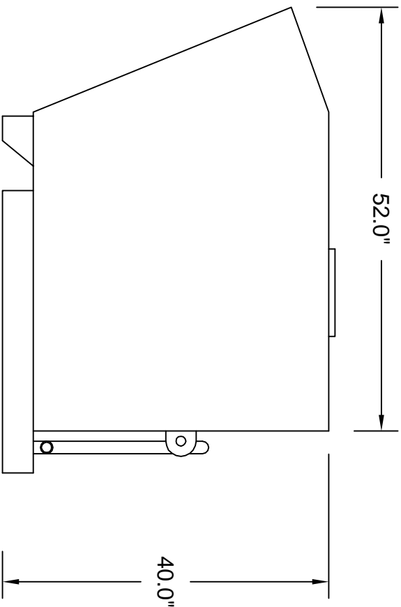
Elevation
