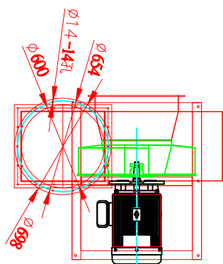
DBN-400 blower
