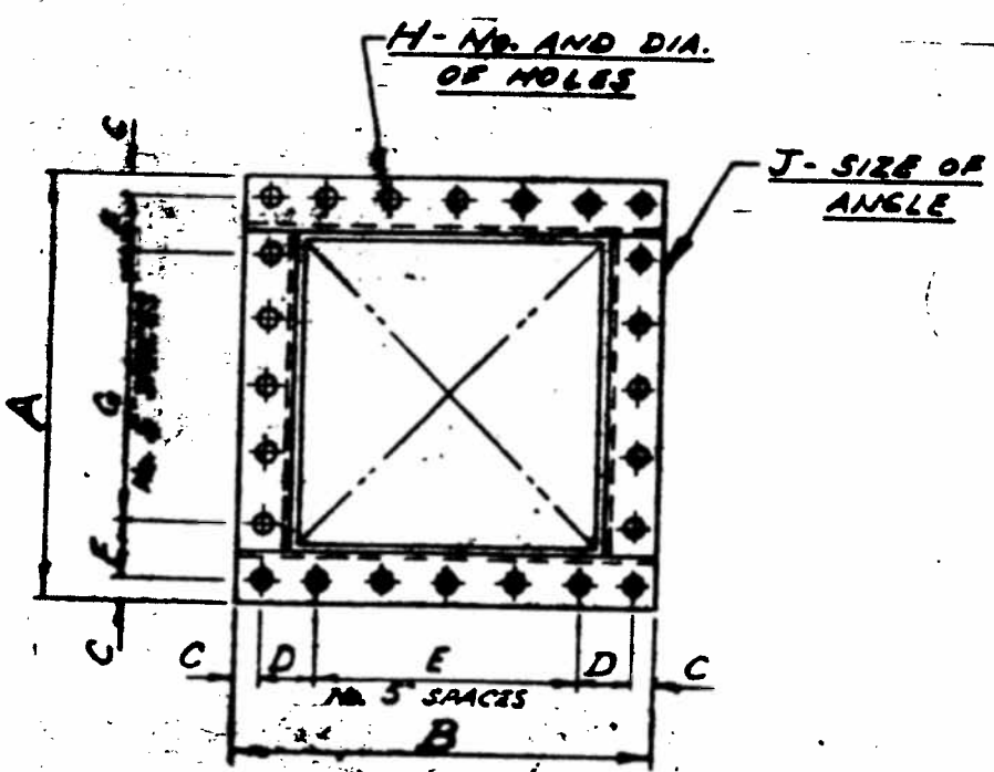
OUTLET FLANGE
