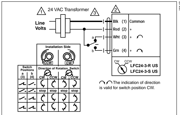
Wiring LFC24-3-R US
