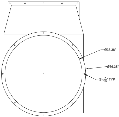
Fan Inlet
